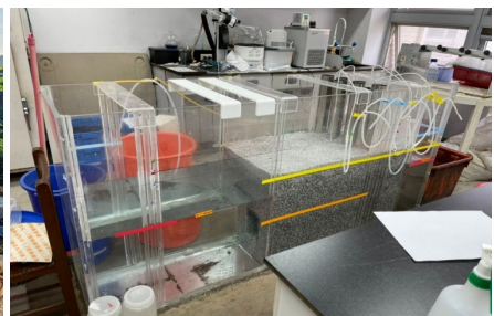
▲反應牆攔截試驗操作實景
